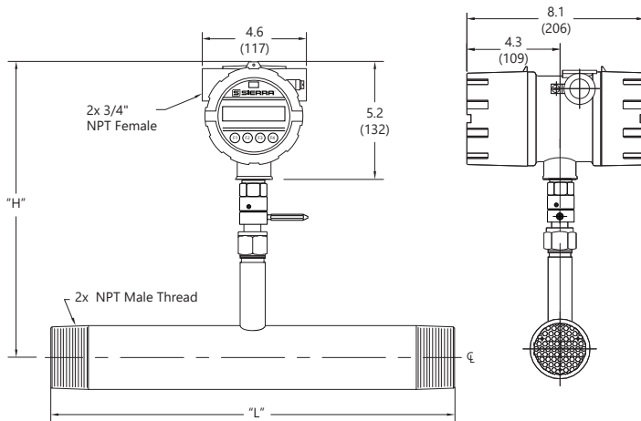
745i Inline Meter - NPT
