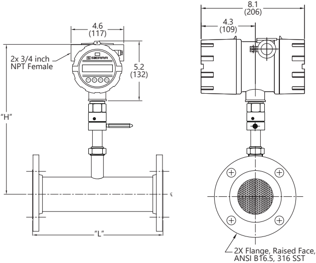
Inline Meter - 150 lb Flange
