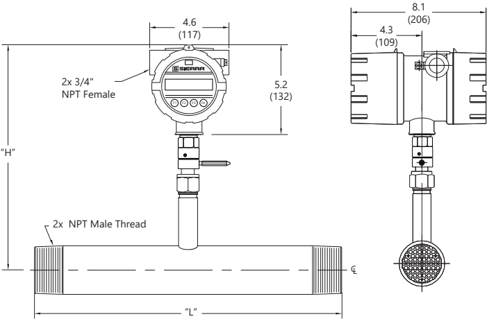
Inline Meter - NPT
