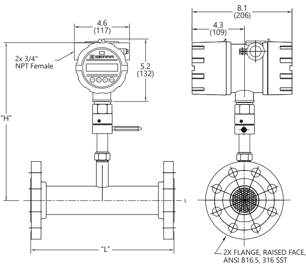
Inline Meter - 300 lb Flange
