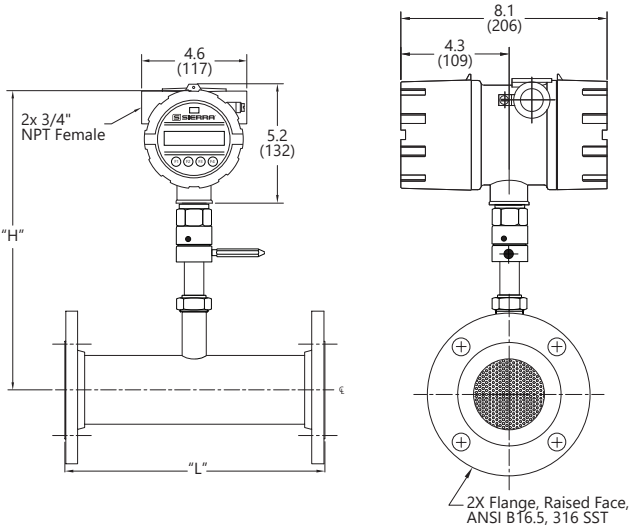
Inline Meter - 150 lb Flange
